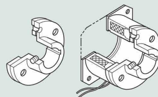
Armature type-1 112[11]
