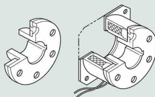
Armature type-2 112[12]
