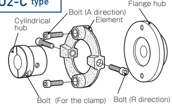
02-C type
