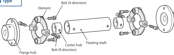
0G type
