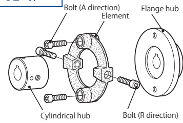
02 type
