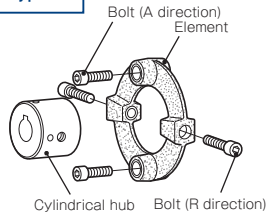
01 type
