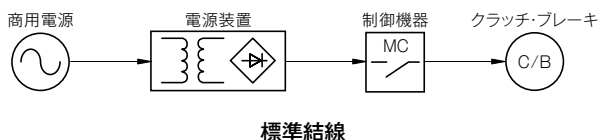
標準結線
