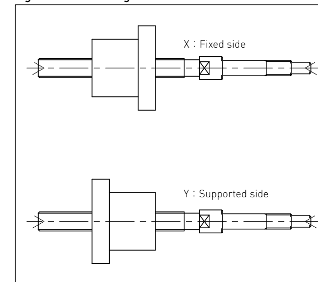
Fig. A-23 : Nut Flange direction
