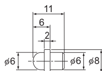
NP6×5 type
